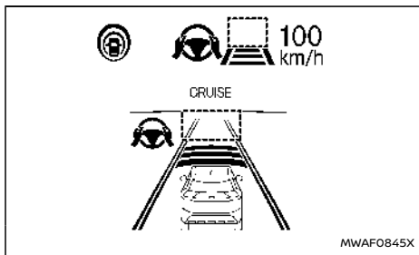
Systemeinstellungsdisplay – kein vorausfahrendes Fahrzeug erfasst*
